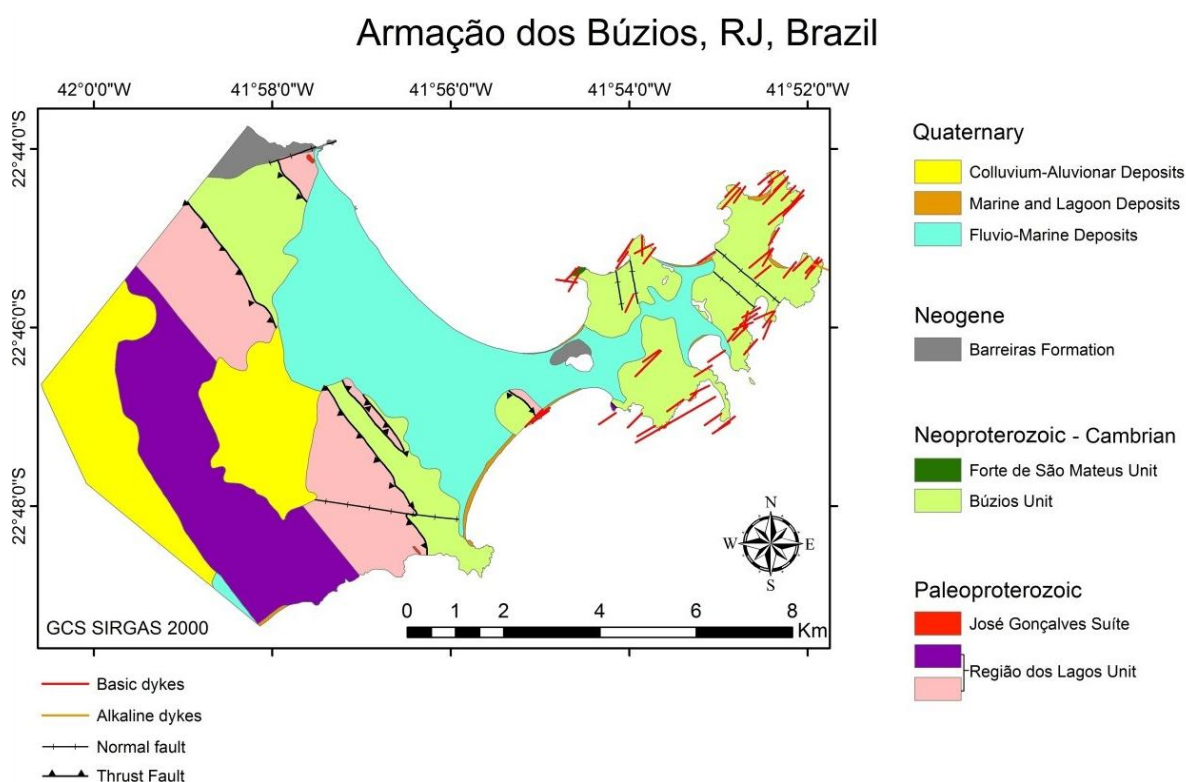
Figure 2 – Geological map of Armação dos Búzios
